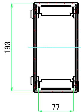
A-A (1:5)
